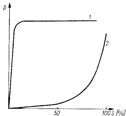
Zależność stopnia polimeryzacji od stopnia konwersji dla polimeryzacji łańcuchowej (krzywa 1) i stopniowej (krzywa 2)
